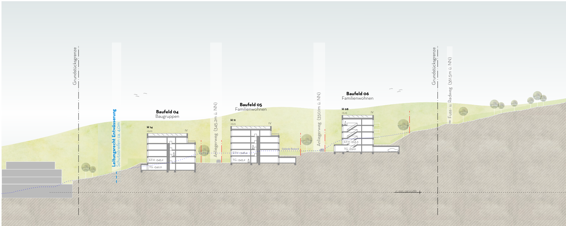
Schnitt A-A
